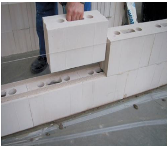
Figura 10 - Bloco sílica-cálcario
