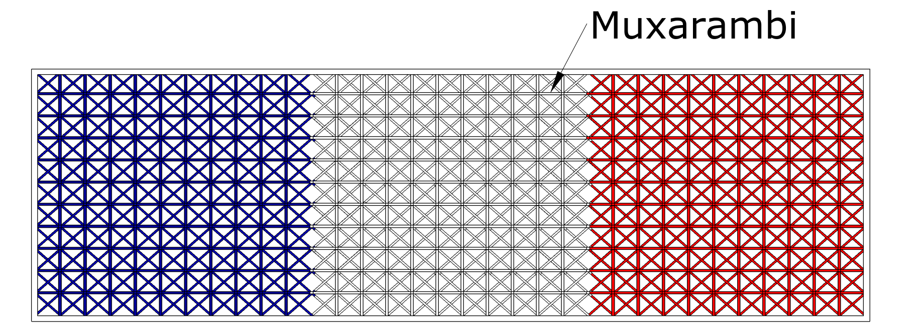
Det. 4 Elemento Fachada Vista Frontal esc.: 1:50
