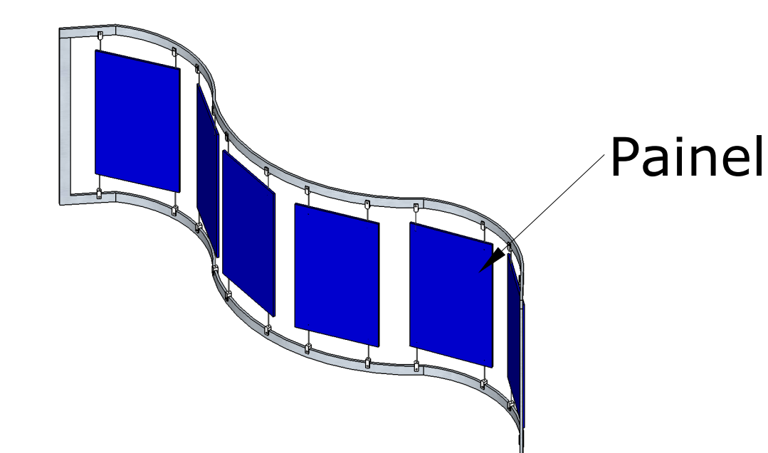
Det. 2 Painel de Exposição - Perspectiva esc.: 1:50
